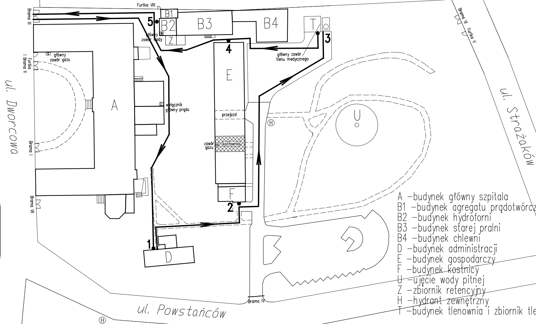
Plan patrolu nocnego Szpitala Chorób Płuc im. św. Józefa w Pilchowicach
